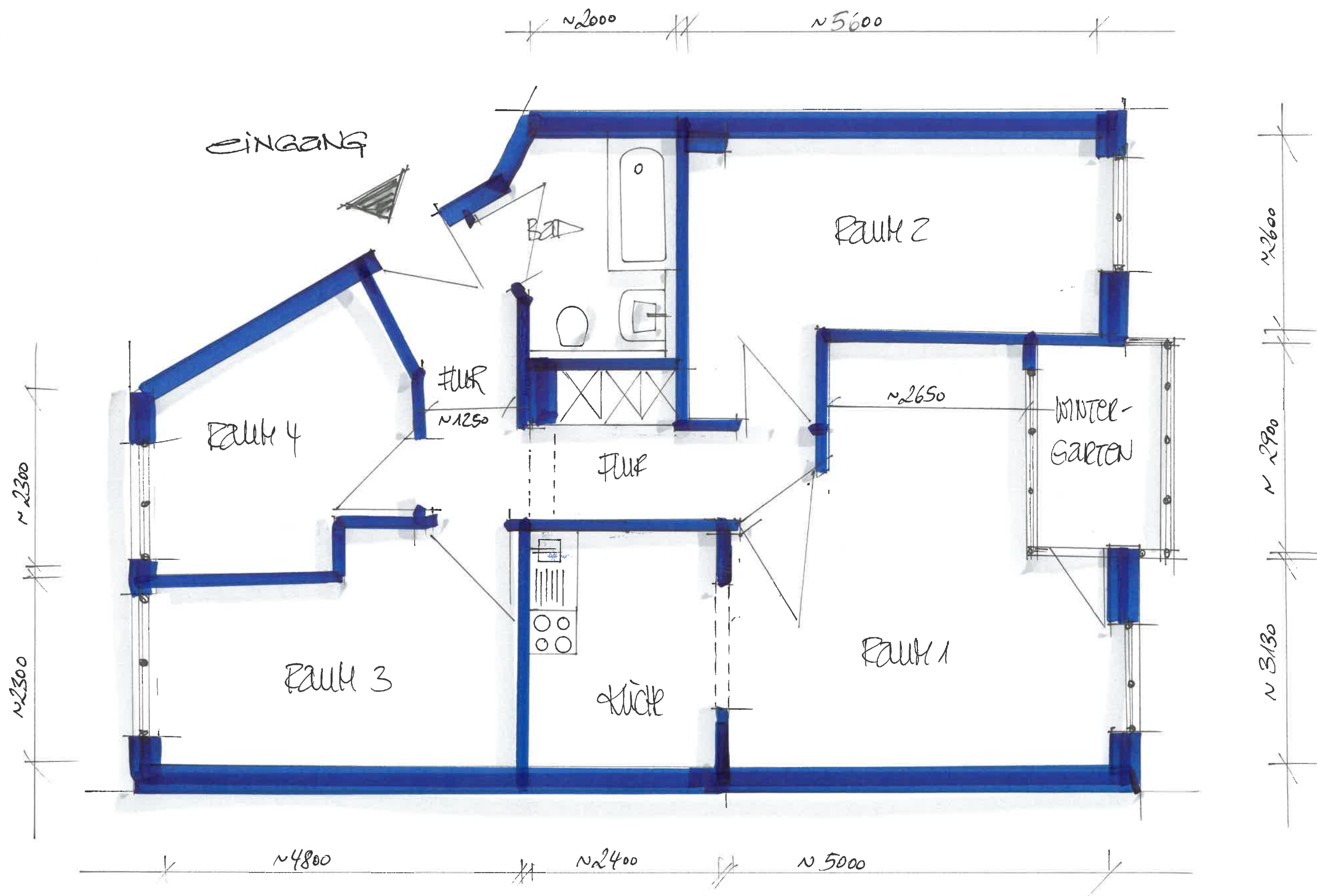
GRUNDRISS 1:50 VE 212.015
